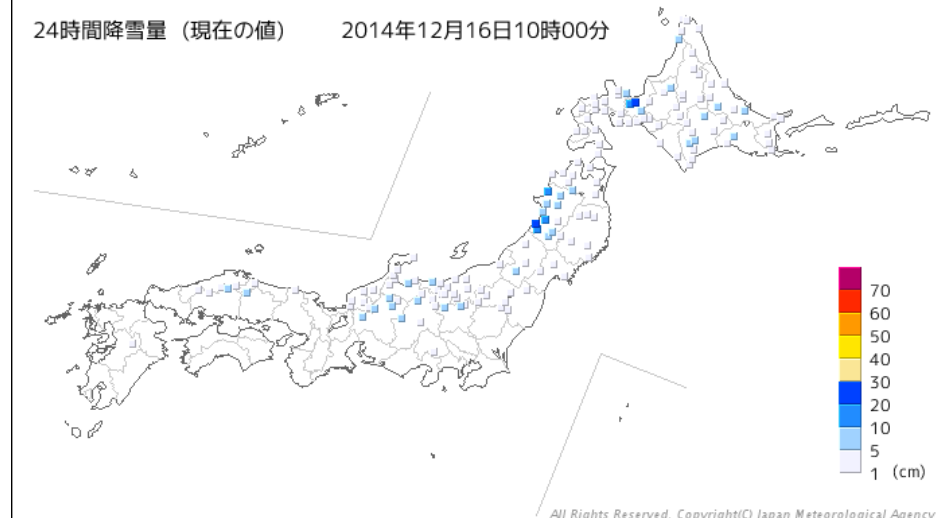
24時間降雪量 10時00分の値
