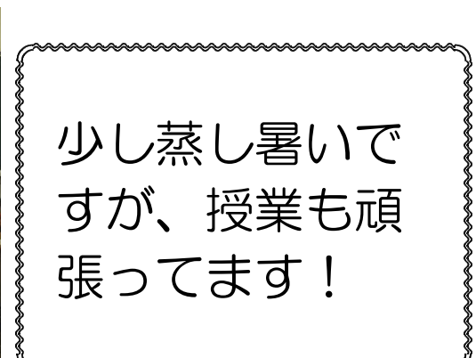
( あかつき )
